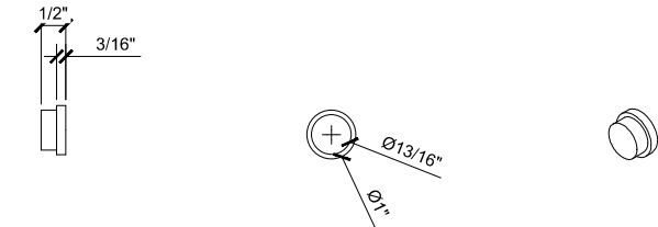
G PLECAP RUBY END CAPS RUBY SLIDING DOORS (XO) SCALE: 6"=1'-0"
